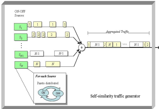
그림 1 자기유사성 트래픽 생성기 모델 Figure 1. Model of self-similar traffic generator
