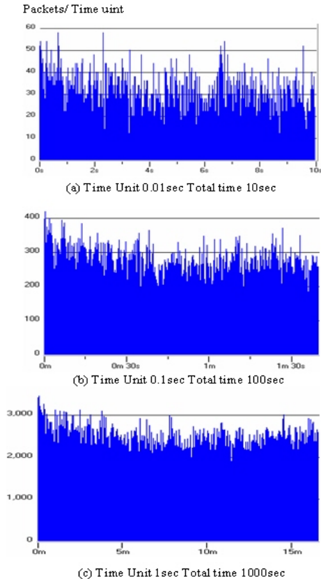
그림 5 시간 척도에 대한 설계된 자기유사성 트래픽 특성 Figure 5. Characteristic of designed self-similar traffic under time scale
