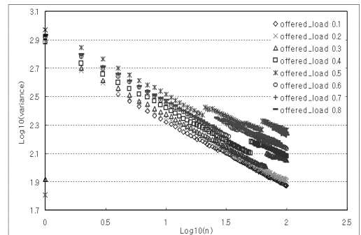
그림 11. 입력 부하에 따른 VT plot Figure 11. VT plot of the offered load
