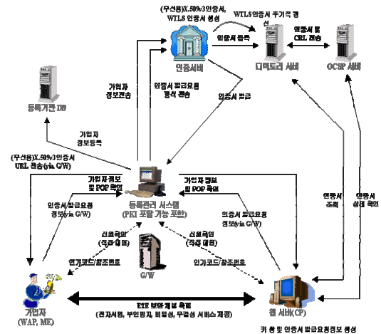
그림 1. 무선 PKI 구성도
