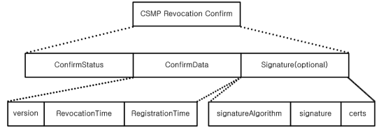
그림 4. CSMP Revocation Confirm 구조도
