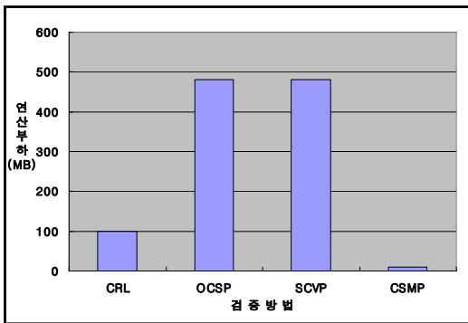
그림 17. 검증자의 연산부하
