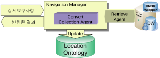
그림 10. Navigation Manager
