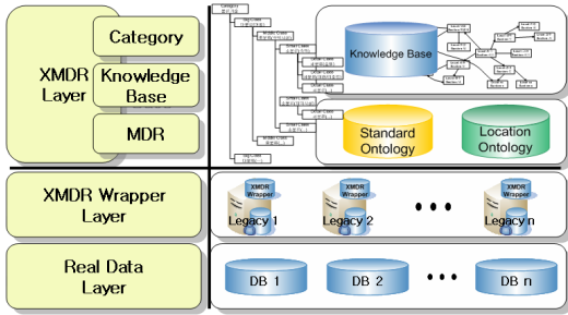
그림 1. XMDR 모델
