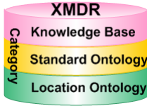
그림 3. XMDR의 개념도
