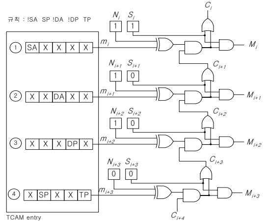
그림 7. nTCAM 구조
