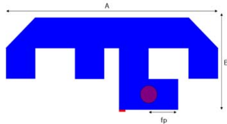
그림 1(a). 설계된 안테나 구조
