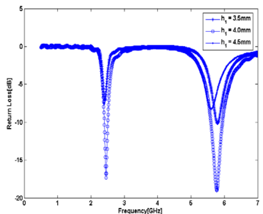
그림 7. 공기층의 두께 h1 변화에 따른 반사계수
