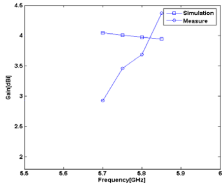
(b) 5.8GHz 대역의 이득 비교
