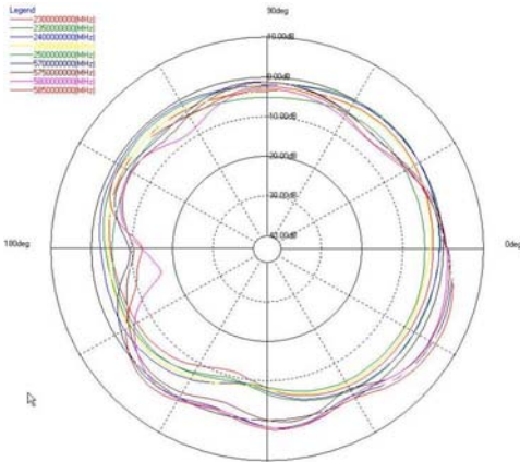
그림 13(a). Azimuth 방사패턴
