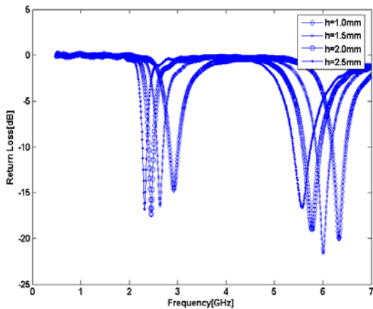
그림 4. 높이 h 변화에 따른 반사계수
