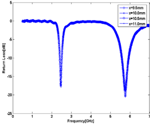
그림 3. 너비 x 변화에 따른 반사계수
