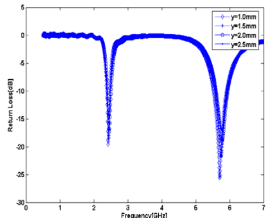
그림 2. 길이 y 변화에 따른 반사계수
