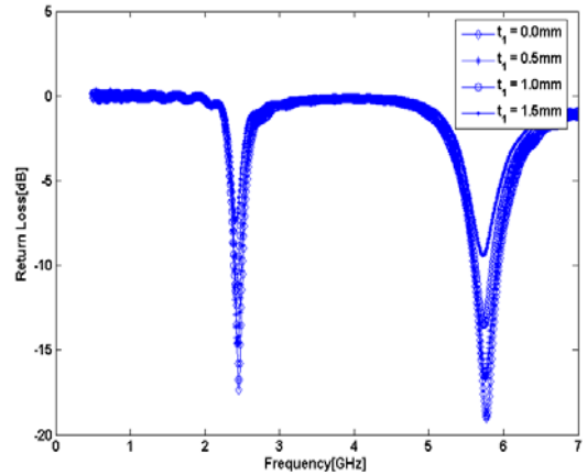
그림 5. 위치 t1 변화에 따른 반사계수
