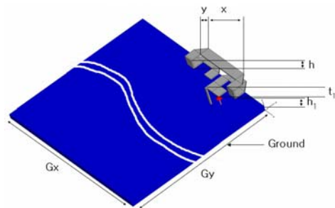
그림 1(c). 설계 안테나의 3차원 구조도
