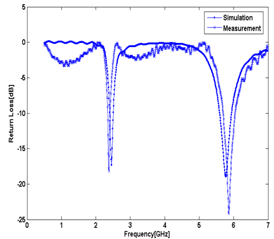
그림 12. 시뮬레이션과 측정 값의 반사계수 비교
