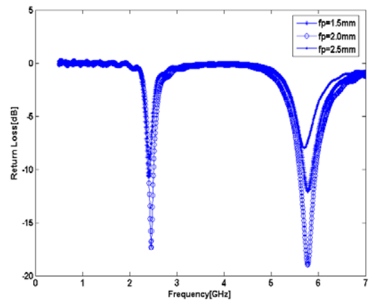
그림 6. 급전 위치 fp 변화에 따른 반사계수
