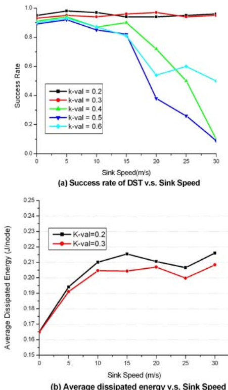
Fig.9. Robustness of the DST
