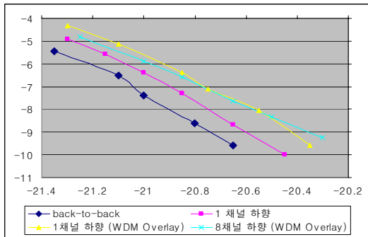
그림 9. WDM 기반 TDM-PON 구조 이용 시 하향 전송실험 결과
