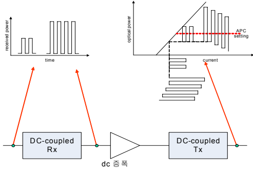
그림 4. 1R 재생에 의한 버스트 모드 송신 광신호
