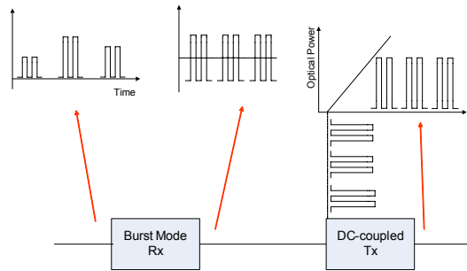
그림 6. 2R 재생에 의한 버스트 모드 송신 광신호
