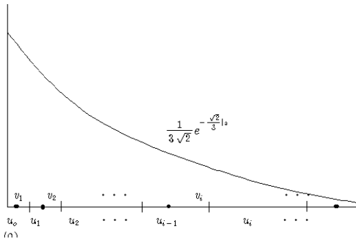
그림 2. Quantile 양자기 Q_{2K} 의 설계. Fig 2. The design of a quantizer Q_{2K}
