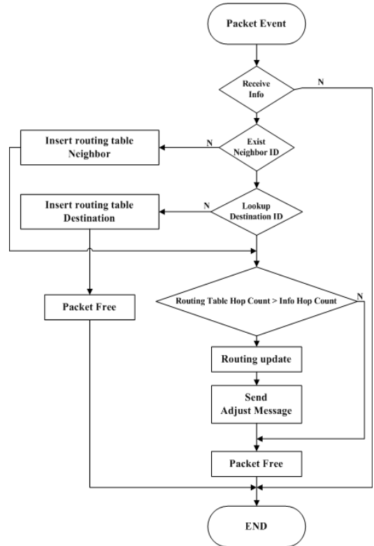
그림 2.6 Info 메시지 처리 절차
