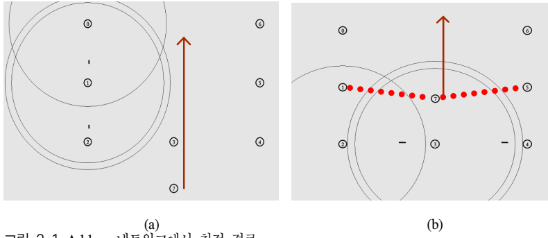
그림 2.1 Ad-hoc 네트워크에서 최적 경로
