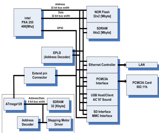
그림 3.16 구현한 임베디드 시스템 블록도
