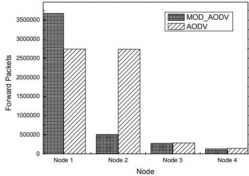
그림 2.10 데이터 포워딩 개수(시나리오 1)
