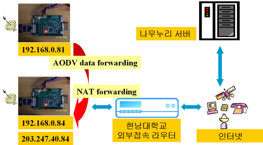
그림 3.9 Ad-hoc 네트워크와 외부 네트워크와의 연동
