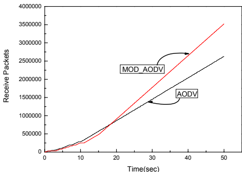
그림 2.9 TCP 패킷 처리량(시나리오 1)
