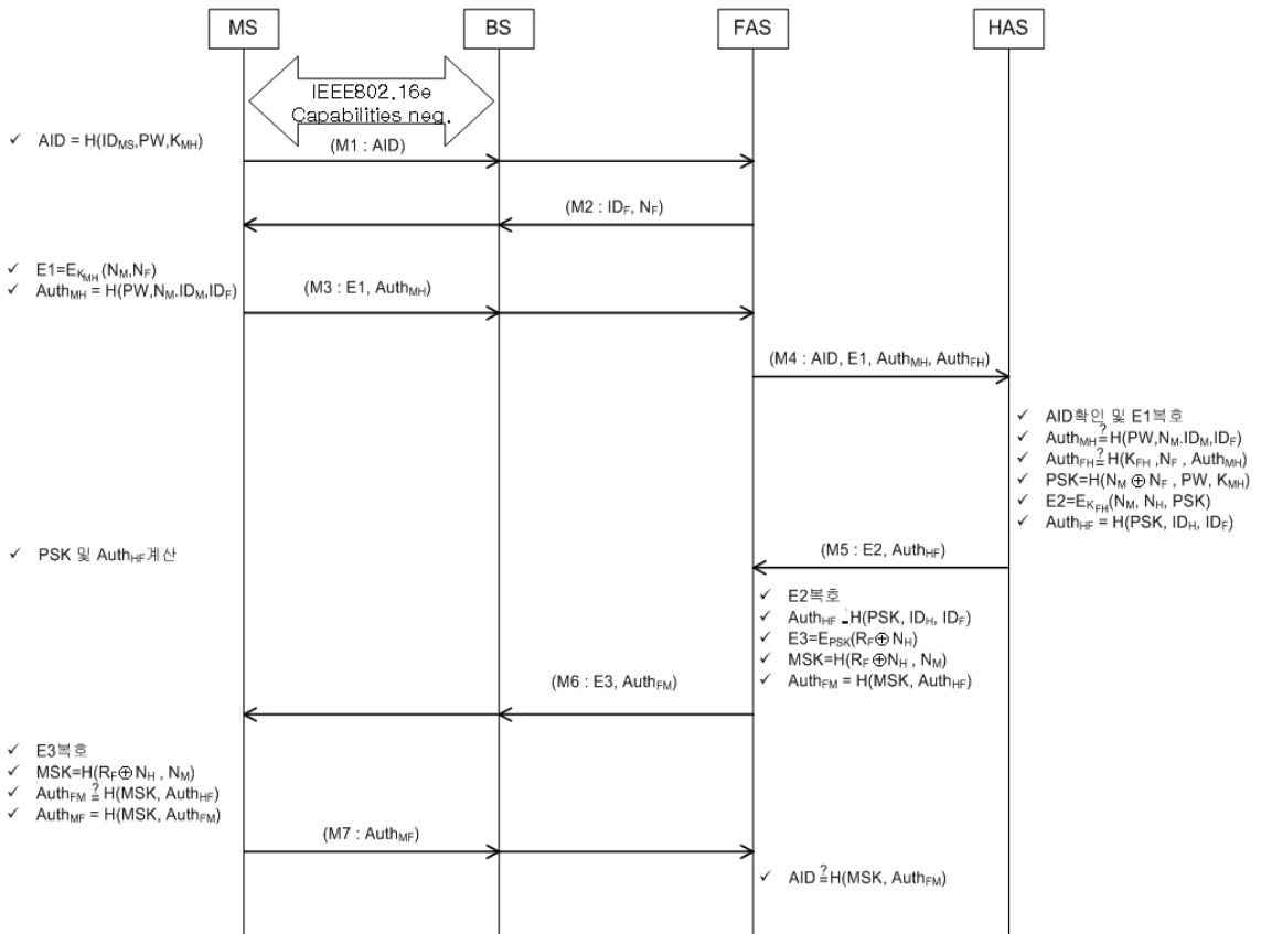
그림 2. 제한된 로밍 인증 및 키 설정 프로토콜
