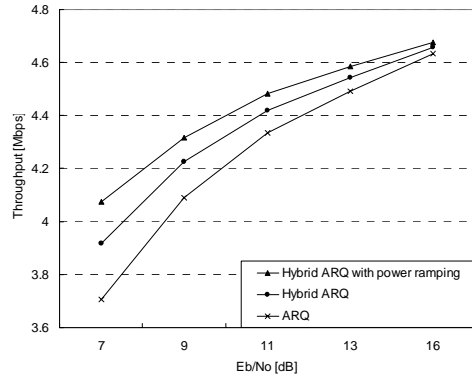
그림 1. 수율과 E_b/N_0 비교 (전력 램핑 단위 크기가=0.5dB) Fig. 1. Throughput versus E_b/N_0 (power ramping step size=0.5dB)
