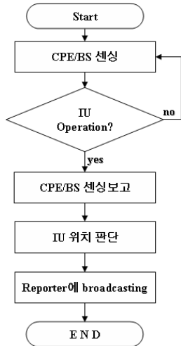
그림 5. A Method의 IU등장 보고절차
