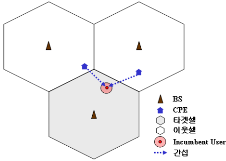
그림 2. 상향링크에서 Incumbent User가 인접 셀의 CR user로부터 받는 간섭
