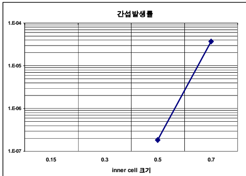
그림 13. Inner Coverage 크기에 따른 간섭발생률
