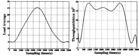
그림 11. 시스템부하평균
