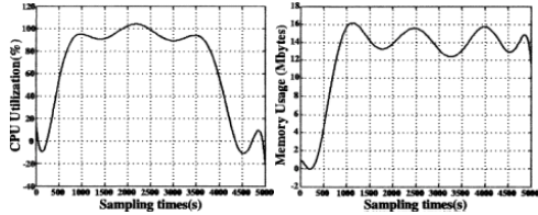
그림 9. CPU 사용률
