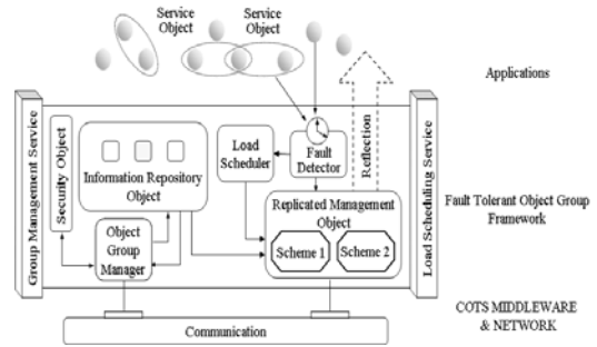
그림 1. FTOG 프레임워크
