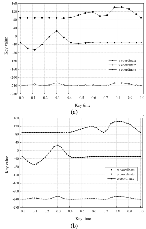
그림 11. (a) 18개 및 (b) 68개의 키를 가지는 Owl 애니메이션의 luleg 변환 노드의 위치 보간기 노드 내에 x, y, z 성분
