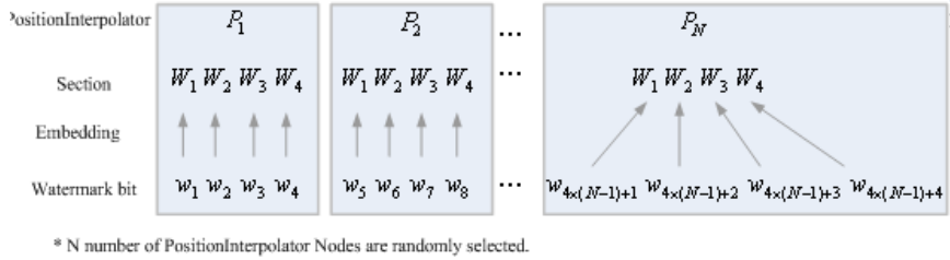
그림 5. N개 선택된 위치보간기 노드에 워터마크 삽입(n=4)
