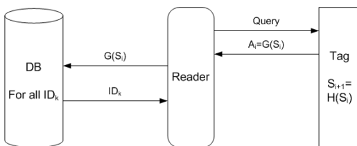
그림 3. 해시 체인 인증 프로토콜
