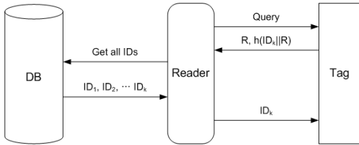
그림 2. 확장된 해시-락 인증 프로토콜
