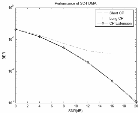
그림 10. 다른 단말의 타이밍 오차 및 지연확산의 영향에 의한 BER 성능
