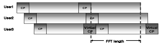
그림 4. 개별 사용자를 위한 보호구간의 확장
