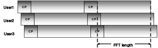
그림 2. 모든 단말이 작은 지연확산 및 타이밍 오차를 가질 때의 보호구간
