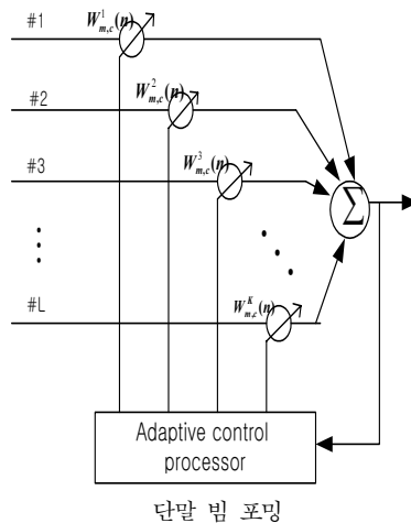
그림 1. 기지국과 단말의 빔형성 시스템 구조
