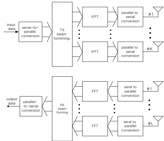
그림 2. 결합 적응적 어레이 안테나 구조
