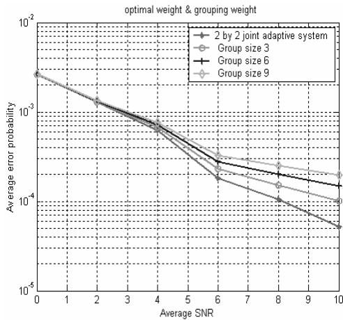
그림 7. 제안된 시스템과의 성능비교
