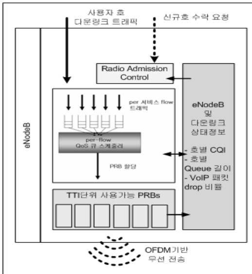
그림 5. 사용자 호별 큐를 가지는 eNodeB의 구조. The eNodeB structure with separate queues for user calls.
