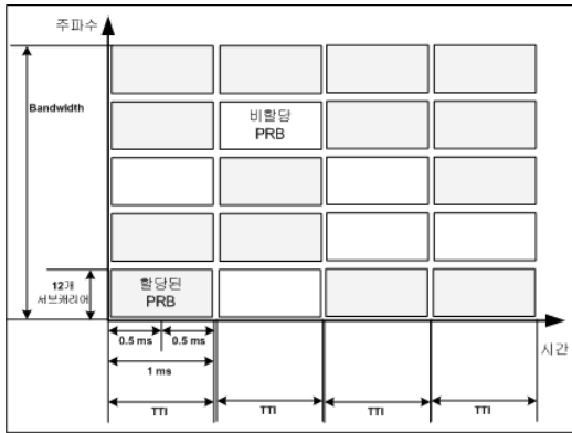
그림 4. eNodeB 전송자원 PRB 구조와 할당. The structure and allocation of the eNodeB transmission resource, PRBs.
