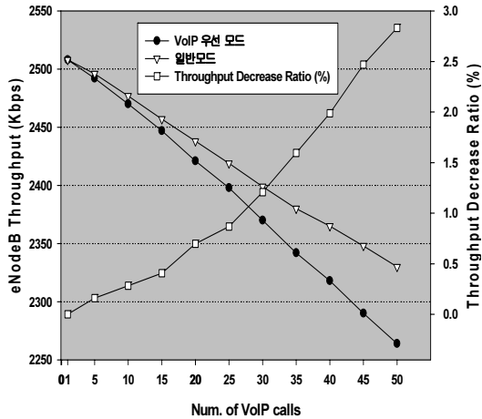
그림 9. VoIP 우선모드와 일반모드에서의 eNodeB throughput 비교와 throughput 감소비율. The eNodeB throughput comparison between the VoIP priority mode and the normal mode, and the plot of the throughput decrease ratio.
