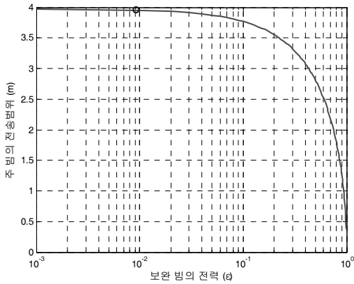
그림 8. 보완 빔 레벨에 따른 AAS 전송 범위
