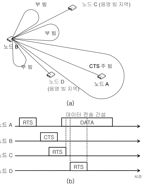
그림 3. 음영 빔 문제
