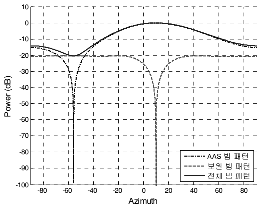
그림 5. 그람-슈미츠 직교화를 이용한 보완 빔 형성 방법의 빔 패턴 DOA=10°, 안테나수=4, 주빔의개수=1
