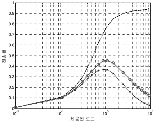
그림 6. 보완 빔을 적용한 시스템 전송률 그래프
