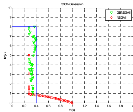
그림 11. 시뮬레이션2의 최종세대 결과
