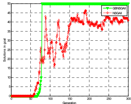
그림 10. 시뮬레이션1의 각 세대별 goal 수렴정도
