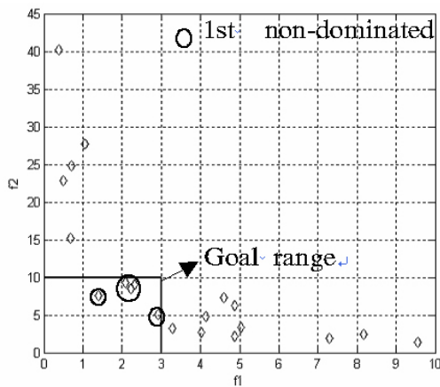
그림 7. 제안한 GBNSGA-II 기반의 1차 비지배 프론트 정렬 예
