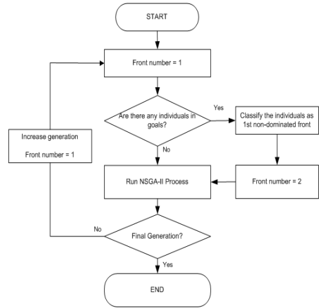
그림 8. GBNSGA-II의 처리 과정
