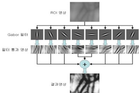
그림 6. 8방향 Gabor 필터링 및 결과영상
