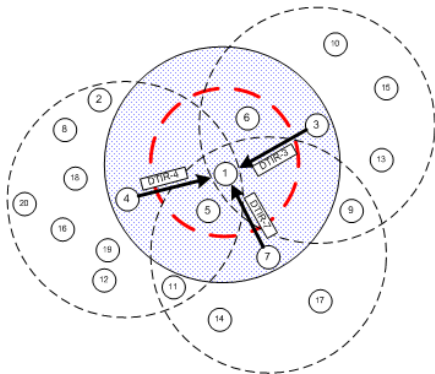
(b) DTIR 패킷의 전송.
