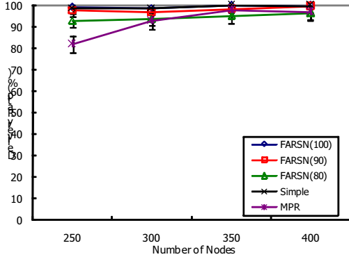
그림 7. 각 flooding 기법의 평균패킷수신비율.
