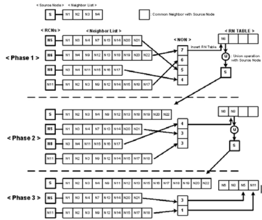
그림 6. 재전송 노드의 선정 과정.
