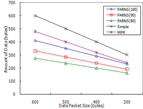
그림 11. 각 노드에서의 데이터 발생량.
