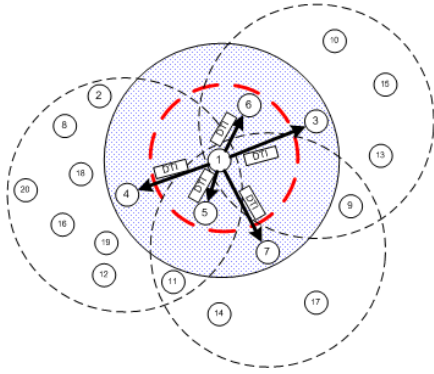
(a) DTI 패킷의 전송.
