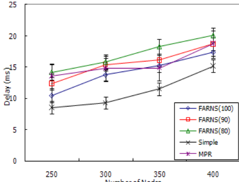
그림 10. 각 flooding 기법의 평균지연.
