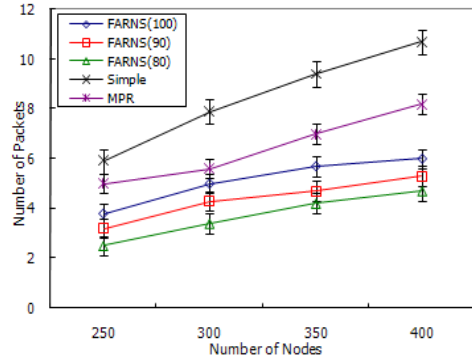
그림 9. 각 flooding 기법의 평균중복패킷의 수.
