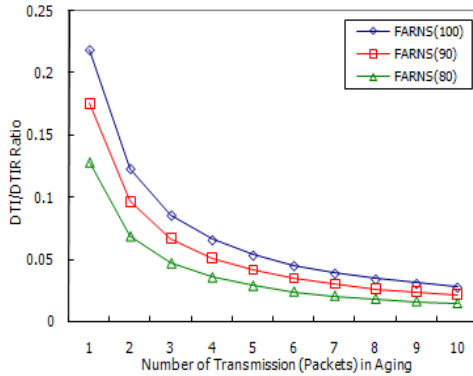
그림 12. Aging 사용시의 DTI와 DITR 패킷의 오버헤드 비율
