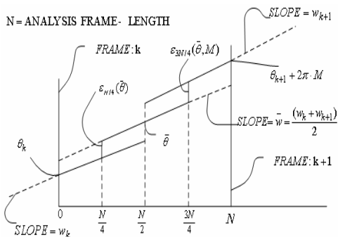
그림 1. N/2 지점의 프레임이 첨가된 위상 관계
