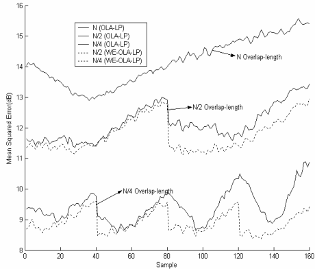
그림 3. 합성 프레임에 따른 각 샘플마다 평균MSE값 (dB) (실선: OLA-LP, 점선: WE-OLA-LP)
