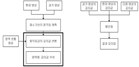
그림 7. 움직임 추정 및 깊이 정보 생성 Fig. 7 Motion estimation and depth map generation
