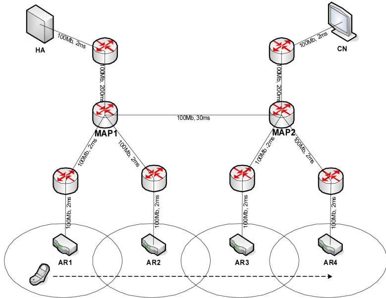
그림 10. 시뮬레이션 네트워크 토폴로지
