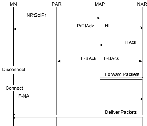
그림 3. MF-HMIPv6 절차
