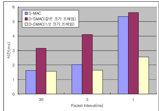
그림 12. S-MAC과 동적 S-MAC의 지연시간 성능 평가
