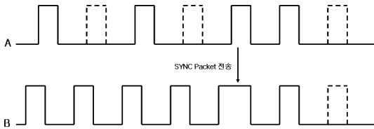
그림 6. 동적 S-MAC 동기화 과정
