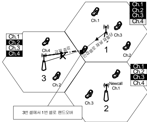
그림 5. 제안하는 Inter-cell DCA 알고리즘의 동작 예(강제종료 시)
