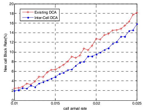
그림 7. 신규호 블록율
