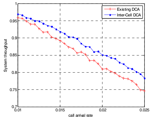
그림 9. 시스템 수율
