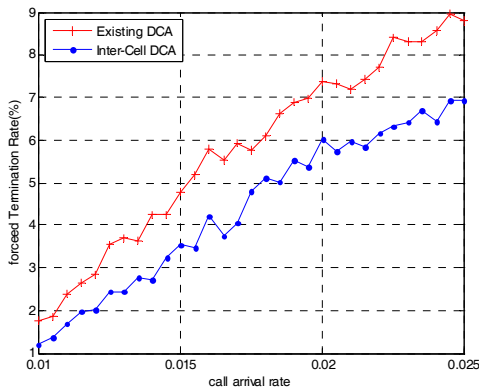
그림 8. 강제 종료율
