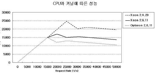
그림 8. CPU와 커널에 따른 성능 Fig. 8. Performance by CPU & kernel
