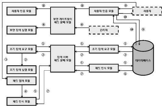
그림 2. 시스템 모듈 세부구조 Fig. 2. System Module architecture
