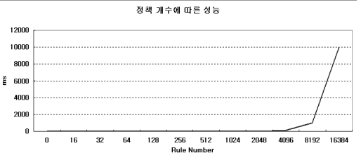
그림 7. 정책 개수에 따른 성능 Fig. 7. Performance by policy count
