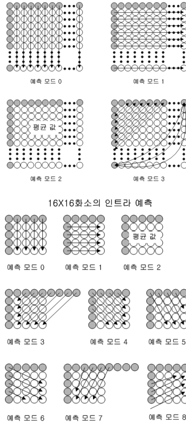
그림 1. H.264/AVC 인트라 부호화의 모드
