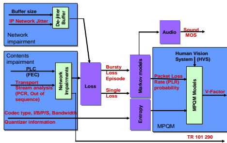
그림 3. V-Factor 측정 모델
