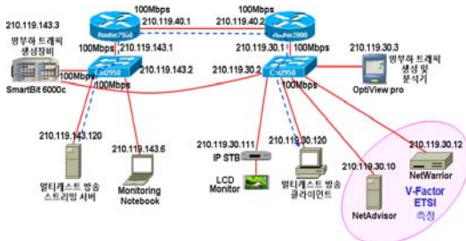
그림 4. 실험실 망의 기본 구성도
