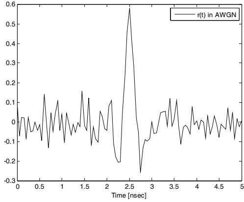
그림 4. AWGN 채널을 통과한 UWB 펄스 Fig. 4. Transmitted UWB pulse over AWGN channel
