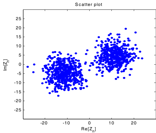
그림 7. CM1을 통과한 수신신호의 산점도 Fig. 7. Scatterplot of UWB pulse over CM1 channel
