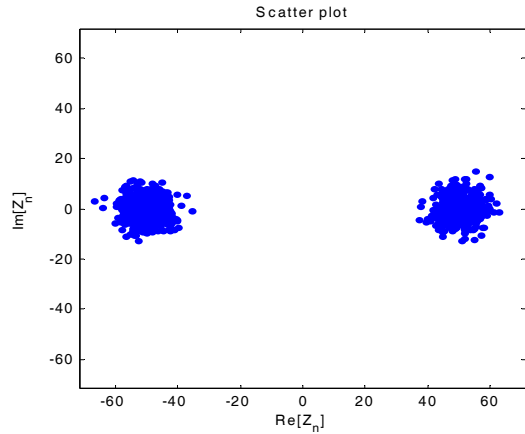
그림 5. AWGN 채널에서 수신펄스의 산점도 Fig. 5. Scatterplot of UWB pulse in AWGN channel
