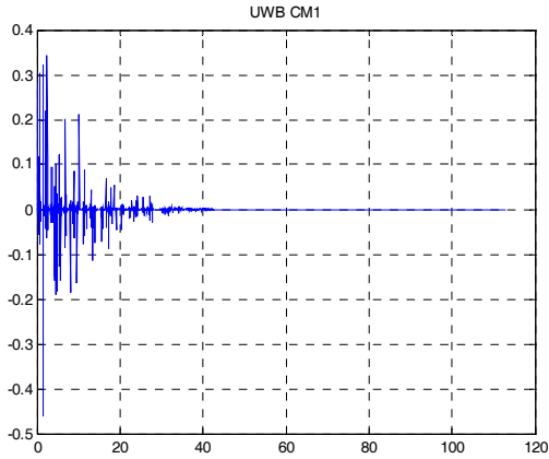
그림 10. CM1 임펄스 응답 h(t) Fig. 10. CM1 impulse response h(t)
