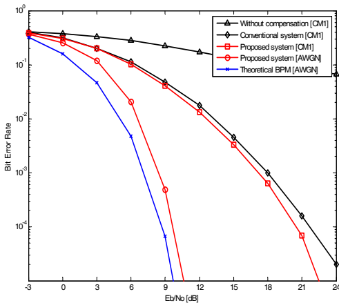
그림 14. BER 성능 비교 Fig. 14. BER performance comparison
