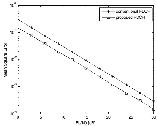
그림 13. MSE 성능 비교 Fig. 13. MSE performance comparison
