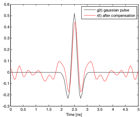
그림 8. 채널 보상한 후의 UWB 펄스 Fig. 8. UWB pulse after channel compensation
