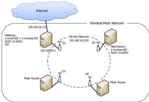
그림 5. WMN 테스트베드 구조
