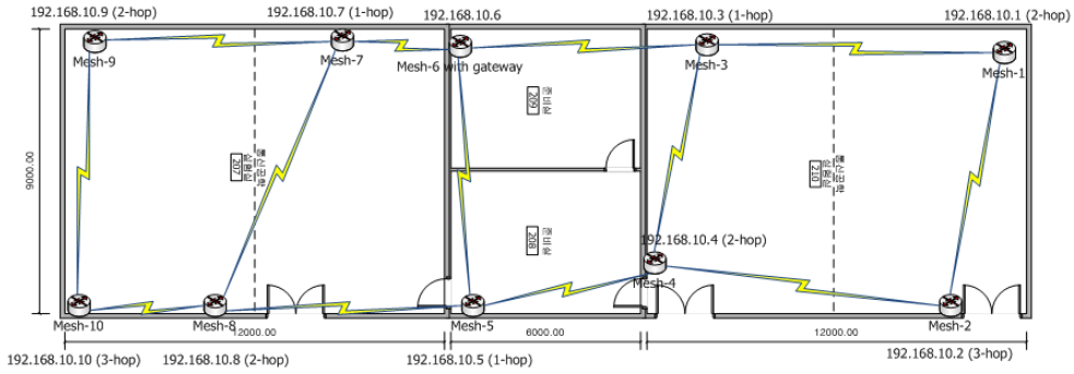
그림 4. 테스트베드 배치도면
