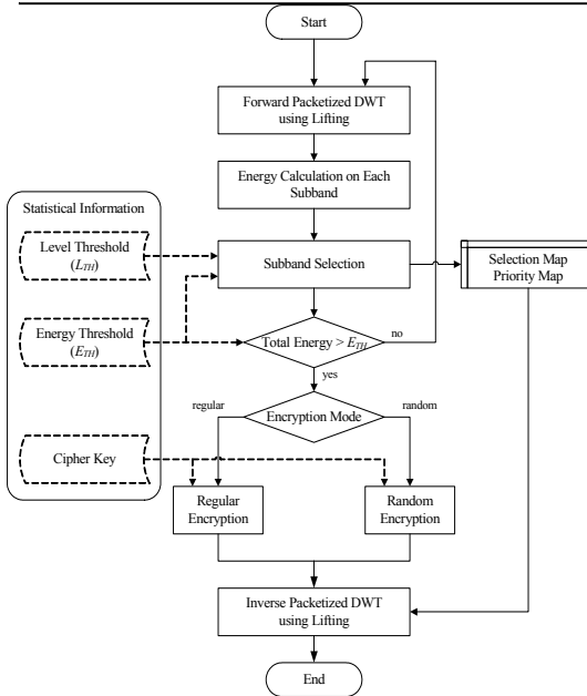
그림 8. 홀로그램 암호화 절차 Fig. 8. Hologram encryption procedure
