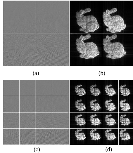
그림 5. 전체 홀로그래프의 국부적 복원 결과 (a) 512×512 크기 (b) 256×256 크기 Fig. 5. Reconstructed objects in local regions, (a) 512×512 size, (b) 256×256 size
