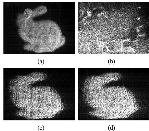
그림 3. 디지털 홀로그래프의 subsampling 후 복원 결과 (a) 원 객체, (b) 1-pixel 단위, (c) 128×128 블록 단위, (d) 64×64 블록 단위의 subsampling Fig. 3. Image example after subsampling digital hologram (a) original 3D object, reconstructed object after sub-sampling by a unit of (b) one pixel, (c) 64×64 block, (d) 128×128 block
