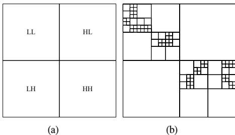
그림 2. DWT에 의한 부대역의 생성 (a) 1 레벨 (b) 5 레벨의 예 Fig. 2. Subband structure example by DWT (a) 1 level (b) 5 level
