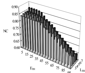
그림 14. 디지털 홀로그램의 암호화 결과 (a) PSNR (b) NC Fig. 14. Encryption result of digital hologram (a) PSNR (b) NC
