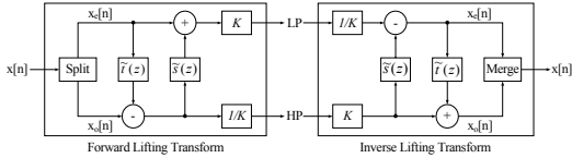
그림 1. 팩토링을 이용한 정방향역방향 리프팅 Fig. 1. Forward/inverse lifting using factoring
