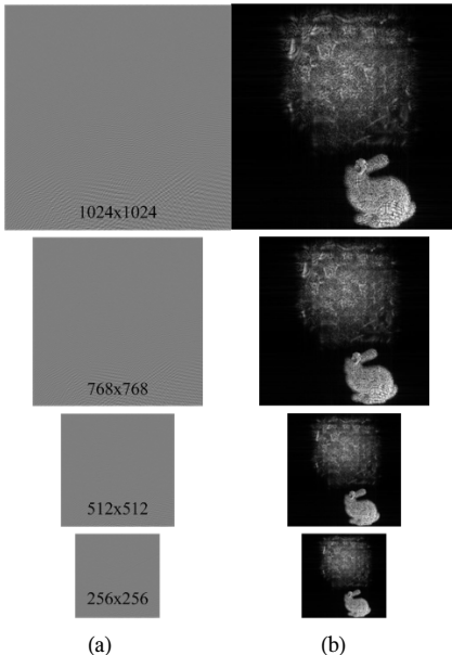
그림 4. Fringe 패턴의 분할을 통한 디지털 홀로그래프의 스케일링 (a) 중심을 기준으로 분할된 fringe 패턴 (b) 분할된 fringe 패턴을 이용한 역 CGH 결과 Fig. 4. Scaling examples using cropping digital hologram (a) cropped holograms, (b) reconstructed objects
