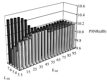
그림 15. 객체의 암호화 결과 (a) NC (b) PSNR Fig. 15. Encryption result of object (a) NC (b) PSNR
