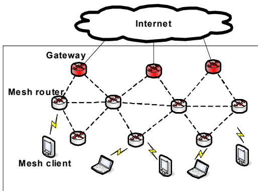
그림 1. 무선 메쉬 네트워크 (WMN)
