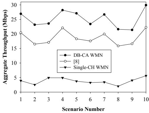
그림 4. 시나리오 번호에 따른 네트워크 성능 (60 MRs)
