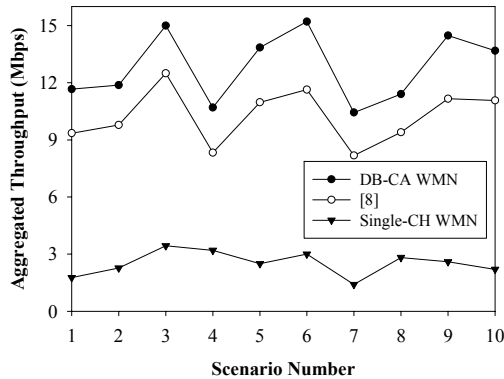
그림 5. 시나리오 번호에 따른 네트워크 성능 (30 MRs)
