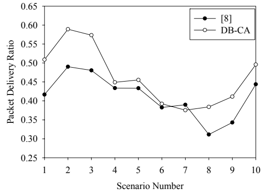
그림 6. 시나리오 번호에 따른 패킷 전달율
