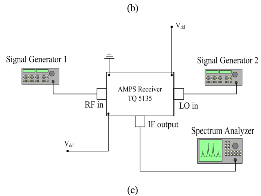
그림 5. TQ5135 AMPS Receiver IC 구동회로 (a) 구동회로도 (b) 제작된 구동회로 (c) 측정도 Fig. 5. The driving circuit for TQ5135 AMPS Receiver IC (a) Driving circuit (b) Fabricated driving circuit (c) Measurement diagram
