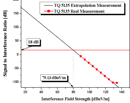
그림 6. 간섭전계강도에 따른 신호대 간섭비 변화의 측정 결과 Fig. 6. Measurement result on the signal to interference ratio in terms of interference field strength
