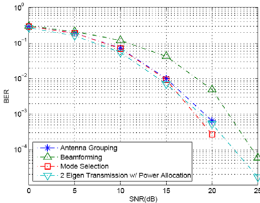
그림 4. IID 채널, BPCU가 8인 4×2 MIMO 시스템에서 평균 BER 성능 (A5 & M1)
