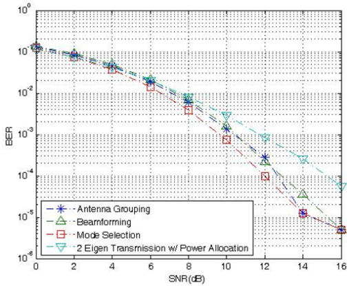
그림 3. IID 채널, BPCU가 4인 4×2 MIMO 시스템에서 평균 BER 성능 (A2 & M1)
