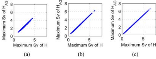
그림 1. 4 \times 2 시스템에서 \lambda_{\max}(H) 와 \lambda_{\max}(H_{AG}) 의 관계 (a) IID 채널, (b) 상관 채널 (angle of departure(AOD): 45°, angular spread(AS): 15°), (c) 상관 채널 (AOD: 45°, AS: 15°)
