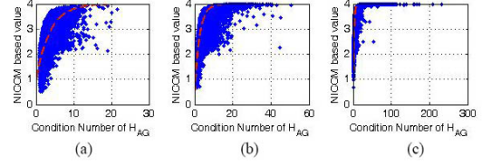
그림 2. 4 \times 2 시스템에서 조건수와 NICCM 값의 관계 (a) IID 채널, (b) 상관 채널 (angle of departure(AOD): 45°, angular spread(AS): 15°), (c) 상관 채널 (AOD: 45°, AS: 15°)
