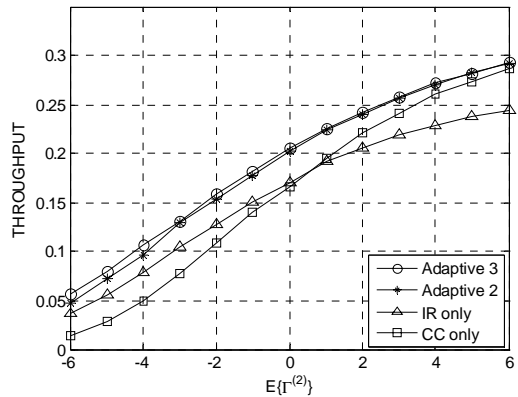
그림 8. M=2, r_1 = 2/3, I_{max} = 3, E\{\Gamma^{(1)}\} = -12 dB일 때, 릴레이의 평균 신호대잡음비에 따른 전송률.
