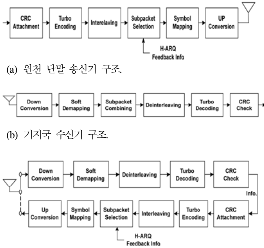
(c) 릴레이 단말의 송수신기 구조.
