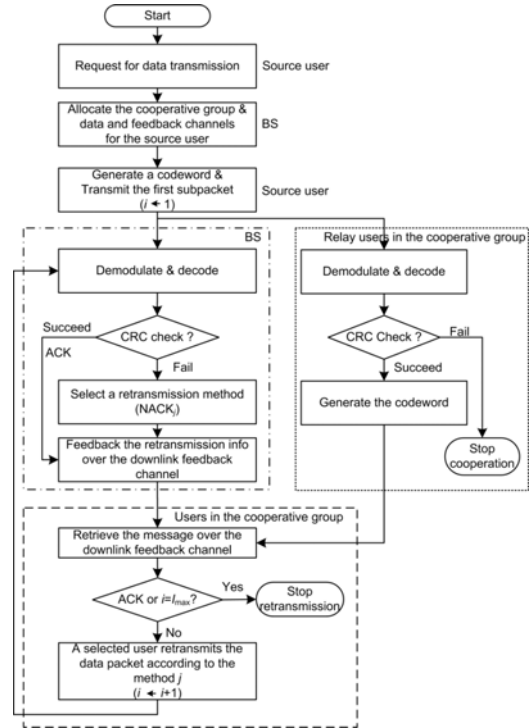
그림 3. 사용자 협력 전송 방식의 순서도.
