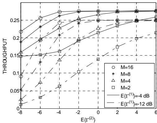
그림 9. 협력 그룹 내 단말 수가 M 이고, r_1 = 1/2 , I_{\max} = 2 일 때 재전송 단말을 선택하는 제안 방법의 전송률.
