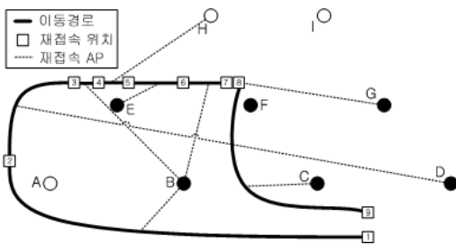
그림 11. Y/T의 이동 경로에서 재접속이 발생한 위치를 표시하고 접속한 해당 AP를 표시
