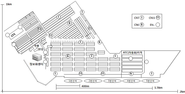
그림 3. 항만에서 조명탑을 중심으로 설치되어 있는 무선 네트워크 인프라의 예
