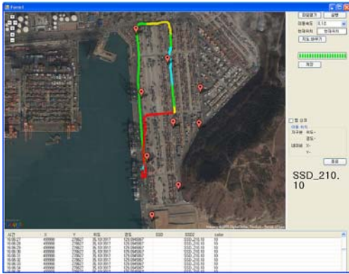
그림 10. Y/T의 이동 경로에 따른 AP 접속현황을 자체 분석 툴을 통해 확인 (측정시간: 15분)
