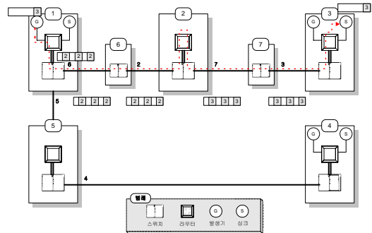
그림 3. 시뮬레이터의 중단간 동작 과정
