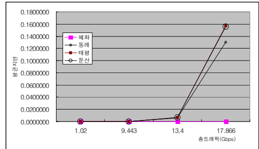
그림 11. 총트래픽량에 따른 노드별 평균지연 비교
