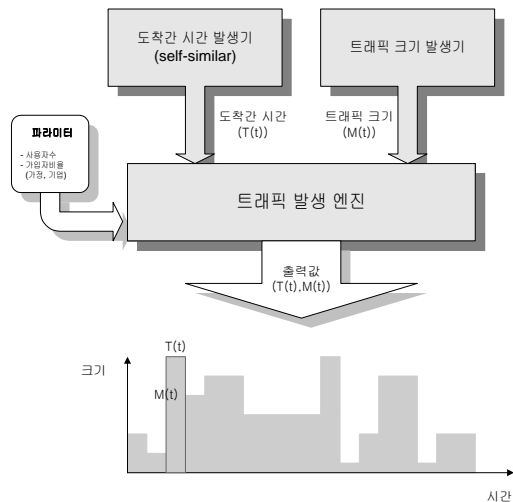
그림 4. 인터넷 트래픽 발생기 구조
