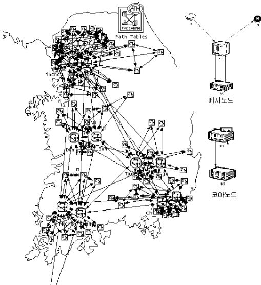
그림 9. 시뮬레이터 외형도
