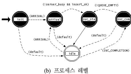
그림 6. OPNET 스위치 구현
