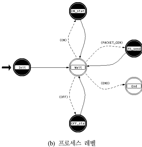
그림 7. 자기 유사 트래픽 발생기 구현
