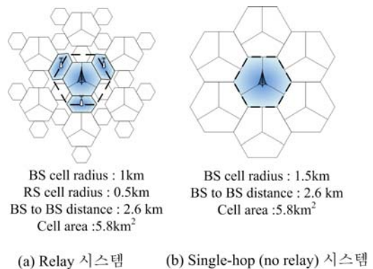
그림 2. 각 시스템의 cell layout
