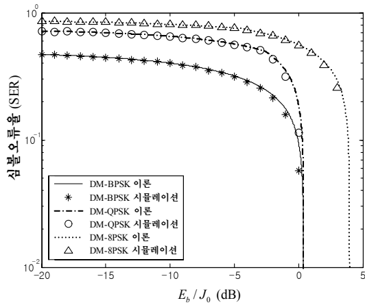
그림 5. 톤 방해전파와 신호에 따른 DM-MPSK의 심볼 오류율 ( G_p = 100 ).
