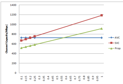
그림 4. 그림 4. AVC, SVC 및 제안된 네트워크 구조에서의 실험 결과, 실험조건 (Punav=10 -4 , L=4, K=300, α=0.6, N 1 =N 2 =N 3 =N 4 =250(상), N=1000(하), a 1 =a 2 =a 3 =a 4 =0.8(상), a=0.8(하), b l ={0.1 0.3 0.5 0.1}(하), R avc,l ={0.128 0.384, 1.5 6}Mbps)
