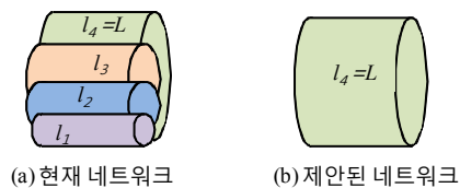
그림 2. 제안된 SVC 전송방식과 이전 방식 비교
