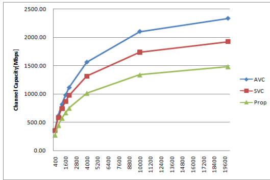
그림 7. AVC, SVC 및 제안된 네트워크 구조에서의 실험 결과, 실험조건(Punav=10-4, L=4, K=300, \alpha=0.6 , N1=N2=N3=N4=N/4 (상), a1=a2=a3=a4=0.8 (상), a=0.8 (하), bl=\{0.1\ 0.3\ 0.5\ 0.1\} (하), Ravc,l=\{0.128\ 0.384,\ 1.5\ 6\} Mbps )
