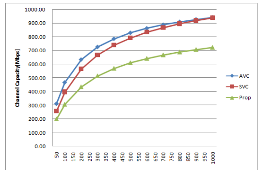
그림 5. AVC, SVC 및 제안된 네트워크 구조에서의 실험 결과, 실험조건(Punav=10 -4 , L=4, α=0.6, N 1 =N 2 =N 3 =N 4 =250(상), N=1000(하), a 1 =a 2 =a 3 =a 4 =0.8(상), a=0.8(하), b l ={0.1 0.3 0.5 0.1}(하), R avc,l ={0.128 0.384, 1.5 6}Mbps)
