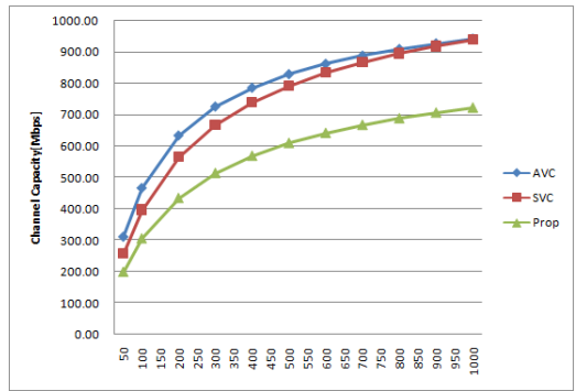
그림 6. AVC, SVC 및 제안된 네트워크 구조에서의 실험 결과, 실험조건(Punav=10-4, L=4, K=300, \alpha=0.6 , N1=N2=N3=N4=250(상), N=1000(하), Ravc,l={0.128 0.384, 1.5 6}Mbps, a1=a2=a3=a4=0.8(상), a=0.8(하), bl={0.1 0.3 0.5 0.1}(하) )
