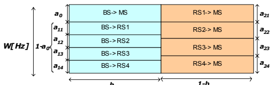
그림 7. 채널 재사용을 하지 않을 때의 프레임 구조 및 SP 비율
