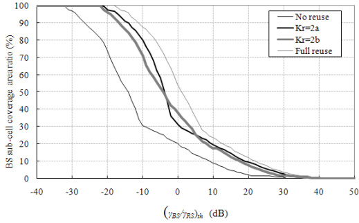
그림 6. (\gamma_{BS}/\gamma_{RS})_{th} 값에 따른 BS sub-cell의 서비스 영역 비율
