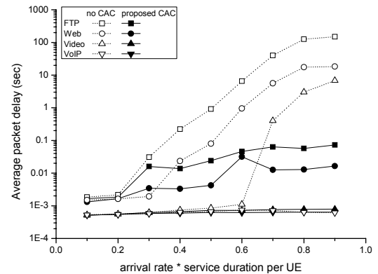
그림 7. 트래픽 혼합비가 1:1:4:4 일 때의 평균 패킷 지연
