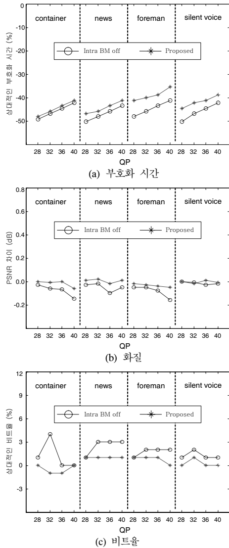
그림 3. 제안된 알고리즘의 성능 비교
