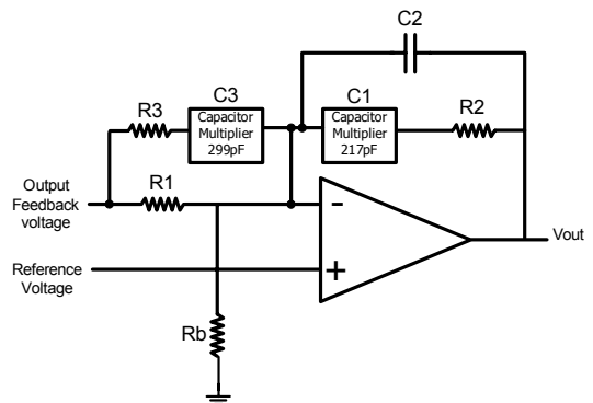
그림 2. 제안된 Type III 오차증폭기 회로 Fig. 2. The proposed type III compensation circuit
