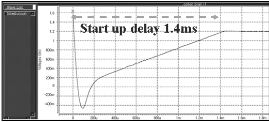
그림 3. 소프트 시동회로 시뮬레이션 Fig. 3. Soft start circuit simulation
