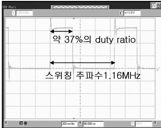
그림 6. 50mA 부하에서의 파워 스위치 구동 전압 출력 Fig. 6. Power switch drive voltage output in 50mA load
