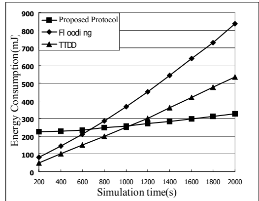
그림 6. 시뮬레이션 시간에 대한 에너지 소모
