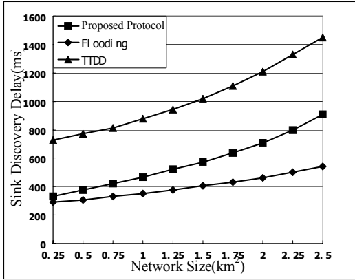
그림 7. 시뮬레이션 시간에 대한 싱크 탐색 딜레이
