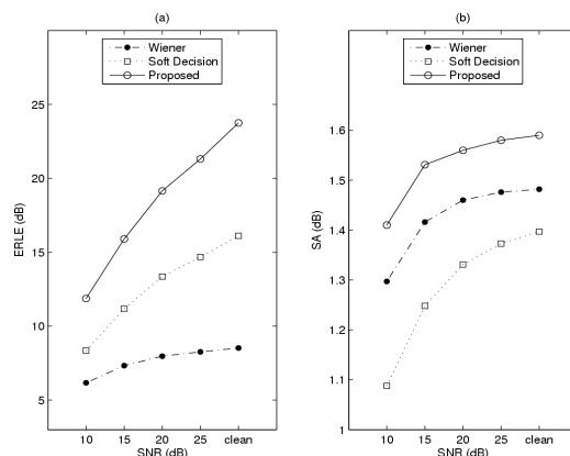
그림 5. 반향 경로가 변화하는 환경에서의 AES 알고리즘의 성능 비교: (a) ERLE 비교 (b) 음성 보존도 (SA) 비교
