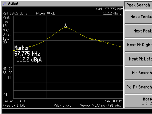
그림 5. 수평으로 구성되어 측정된 58kHz EAS7의 전계강도
