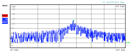
그림 6. B업체에서 측정된 58kHz EAS 시스템의 전계강도
