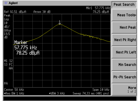
그림 7. 수평으로 구성되어 측정한 58kHz EAS 시스템의 자계강도
