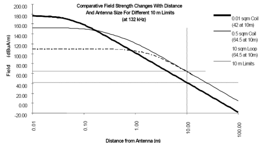
그림 3. 거리에 따른 자계강도의 감쇄량(ERC Report44)
