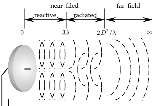
그림 1. 근거리장과 원거리장
