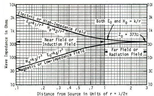
그림 2. 거리에 따른 파동임피던스의 변화 [8]
