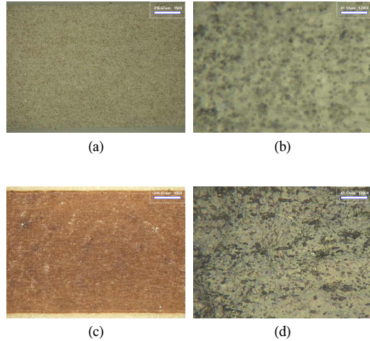
그림 3. ACF 필름 이미지 : (a), (b) 고온 시험 전 ACF 필름(150배율, 1200배율), (c), (d) 고온 시험 후 ACF 필름(150배율, 1200배율)
