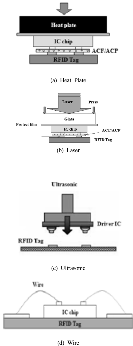
그림 1. RFID 태그 접합 기술
